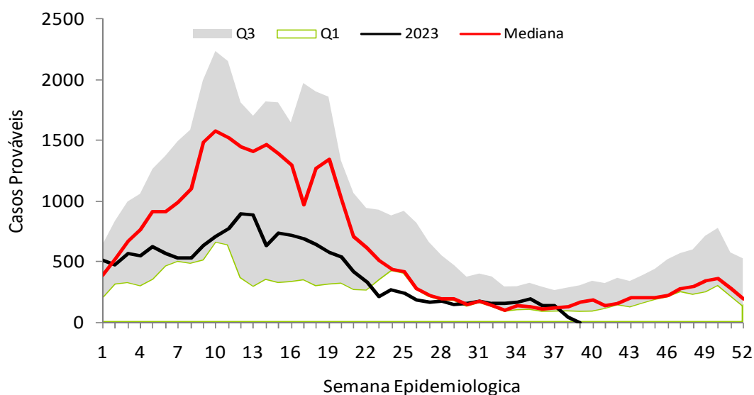
Gráfico 1 – Diagrama de controle da dengue em Goiânia - 2023*
