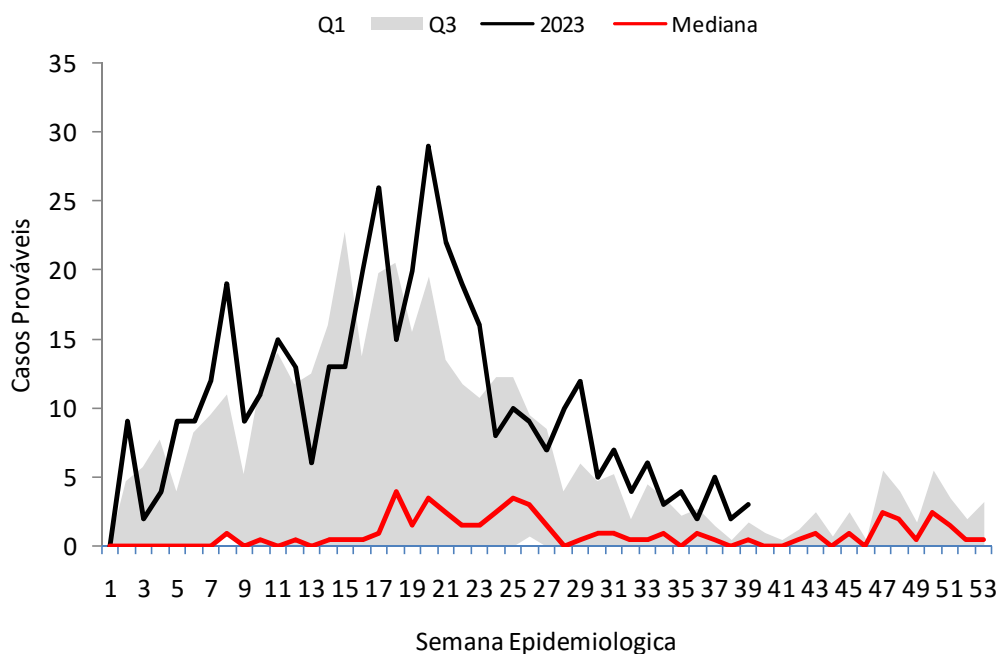
Gráfico 2 – Diagrama de controle de casos prováveis de chikungunya em Goiânia - 2023*
