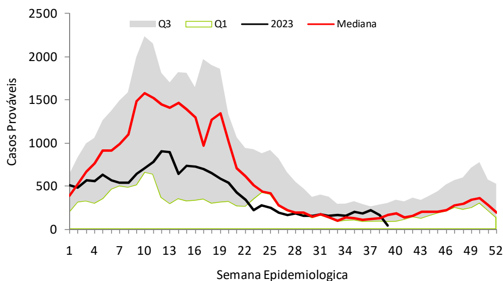
Gráfico 1 – Diagrama de controle de casos prováveis de dengue em Goiânia - 2023*
