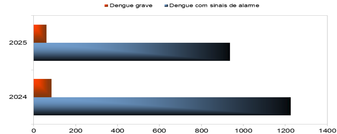
Gráfico 4: Casos confirmados de dengue com sinais de alarme e dengue grave, até SE 24/2025, Goiânia, 2024* e 2025*.
